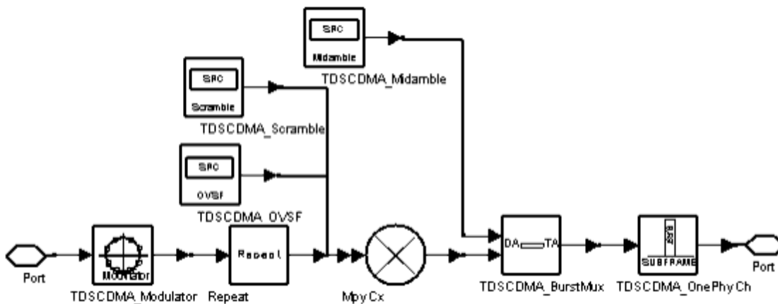
TDSCDMA_PRACH Schematic
